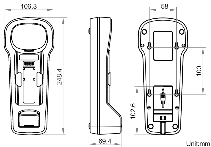
底座：
